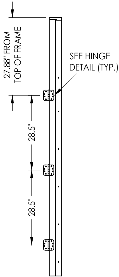
HINGE JAMB
