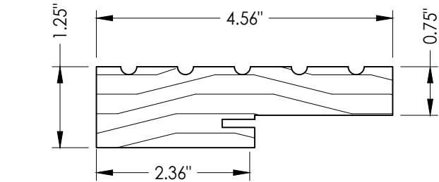
1 WOOD JAMB
