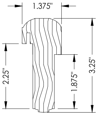
3 ASTRAGAL
